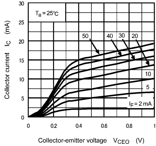
Fig. 11.8 I_C - V_{CEO}
